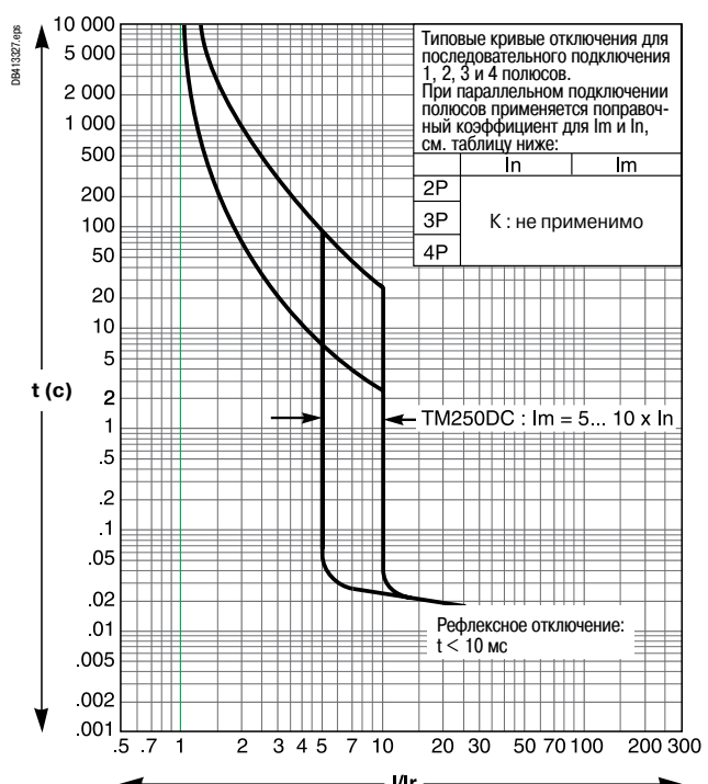
TM250DC
