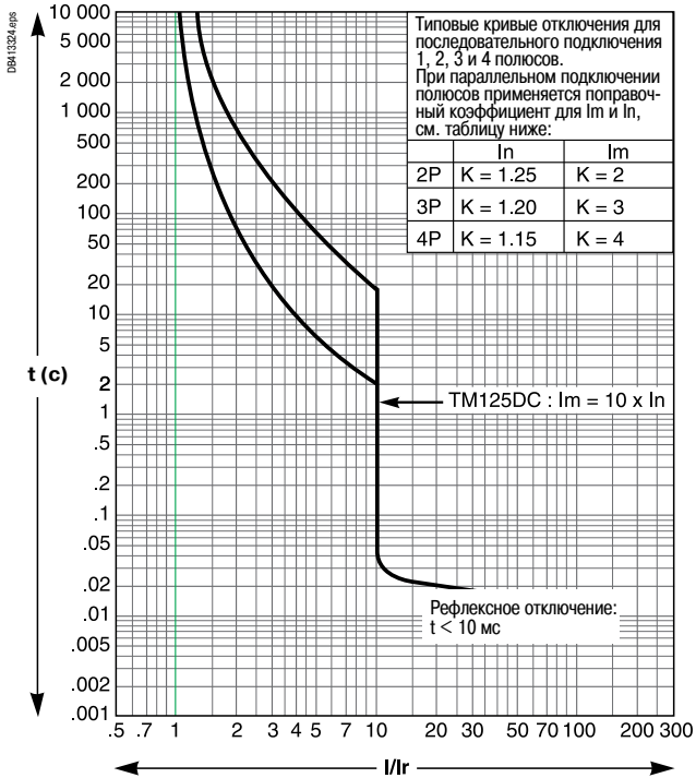
TM125DC
