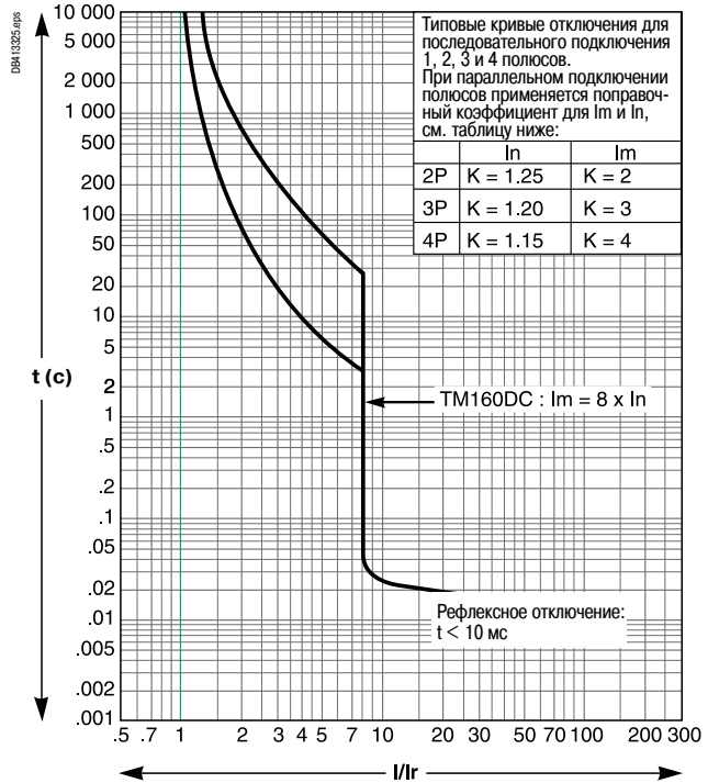
TM160DC
