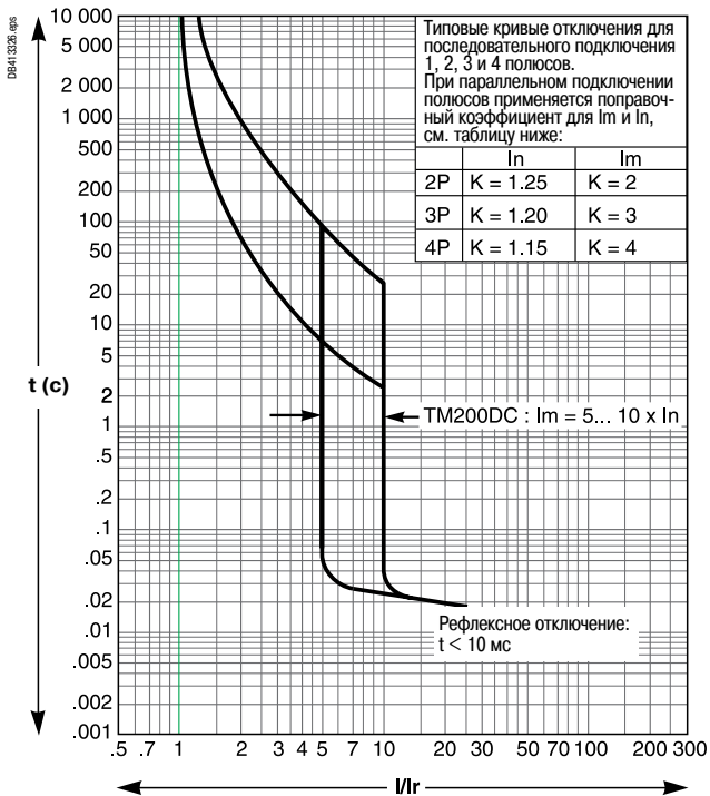
TM200DC
